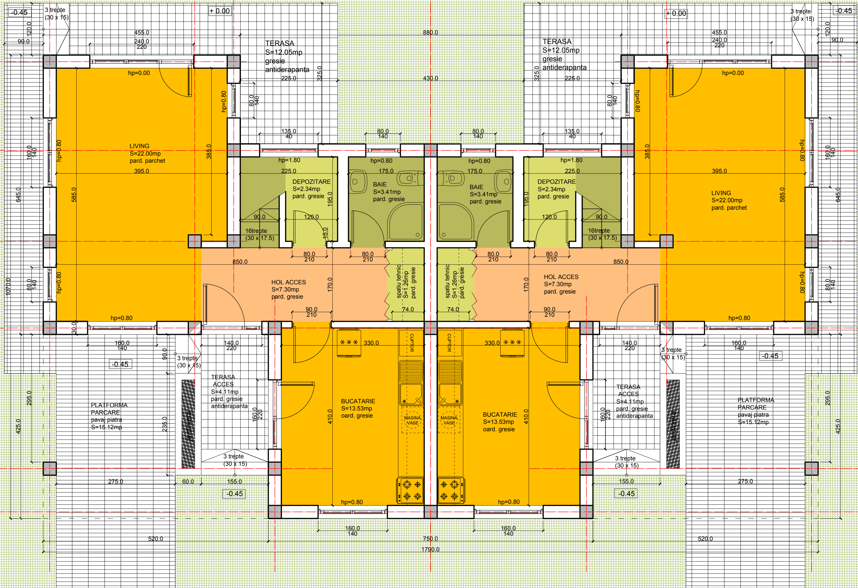
PLAN PARTER suprafata construita = 64,65 mp suprafata utila = 49,84 mp
